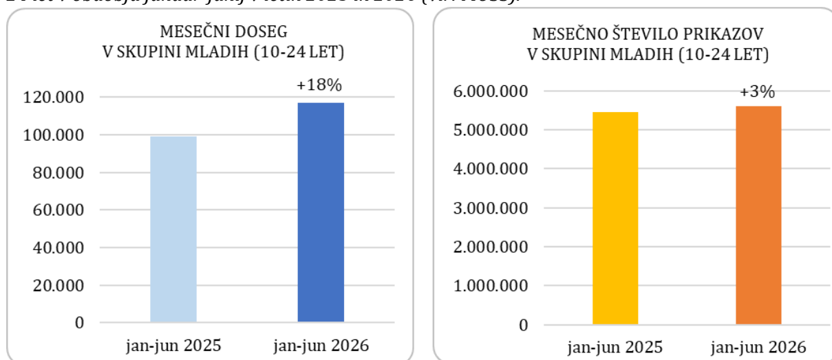
Graf 4.7: Povprečni mesečni doseg in povprečno mesečno število prikazov v ciljni skupini starih 10-24 let v obdobju januar-junij v letih 2025 in 2026 (vir: MOSS).
